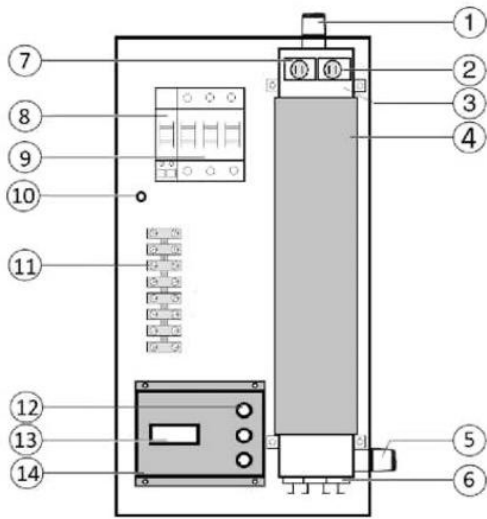
Рис. 2 Функциональные элементы котла AVL Joule AJ-S 3-9 кВт
