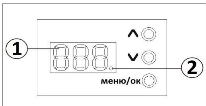
Рис. 13 Панель керування опалювального котла AVL Joule
