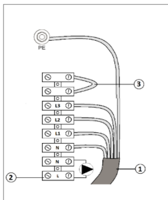
Рис. 11 Подключение к электросети AVL Joule AJ / AJ-S 380 В 3-9 кВт, 3x 400/230 В AC
