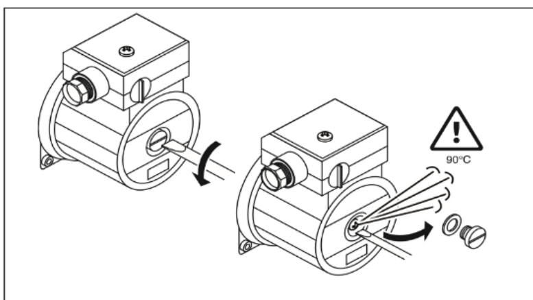
Рис. 8 Послаблення гвинта для спускання повітря та перевірка вільного ходу
