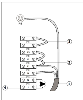
Рис. 9 Підключення до електромережі AVL Joule AJ / AJ-S 3-9 кВт, 1x230 В AC
