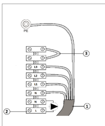
Рис. 11 Підключення до електромережі AVL Joule AJ / AJ-S 380 В 3-9 кВт, 3х 400/230 В AC
