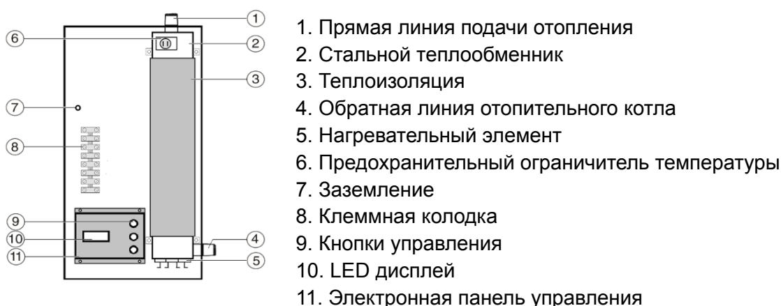
Рис. 1 Функциональные элементы котла AVL Joule AJ 3-9 кВт
