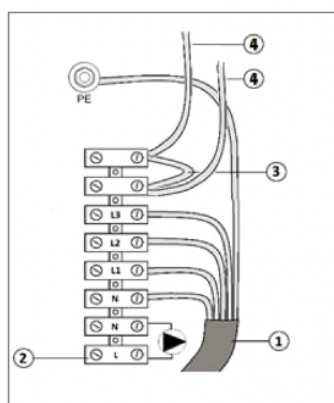
Рис. 12 Підключення до електромережі AVL Joule AJ-WS / AJ-W 380 В 3-9 кВт, 3х 400/230 В AC
