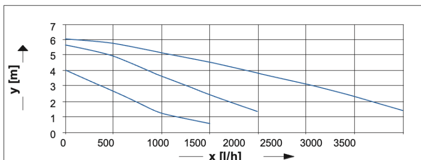
Рис. 16 Напор насоса на примере Wilo RS15/6
