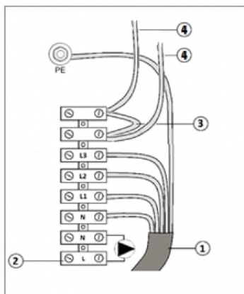
Рис. 12 Подключение к электросети AVL Joule AJ-WS / AJ-W 380 В 3-9 кВт, 3х 400/230 В AC
