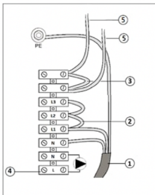
Рис. 10 Подключение к электросети AVL Joule AJ-WS / AJ-W 3-9 кВт, 1x230 В AC
