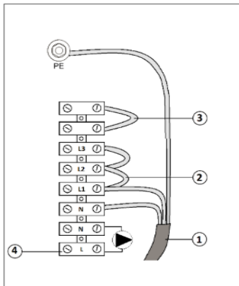
Рис. 9 Подключение к электросети AVL Joule AJ / AJ-S 3-9 кВт, 1x230 В AC
