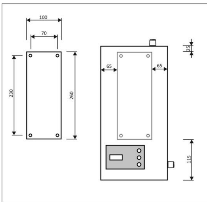
Рис. 6 Розміри отворів для кріплення опалювального котла AVL Joule AJ / AJ-S / AJ-WS / AJ-W
