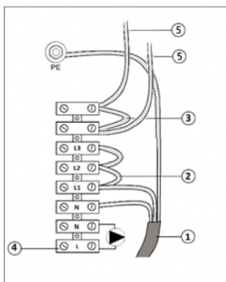
Рис. 10 Підключення до електромережі AVL Joule AJ-WS / AJ-W 3-9 кВт, 1x230 В AC
