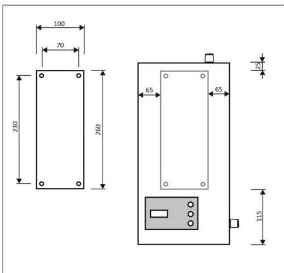
Рис. 6 Размеры отверстий для крепления отопительного котла AVL Joule на стене
