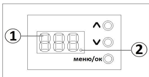
Рис. 13 Панель управления отопительного котла AVL Joule AJ / AJ-S / AJ-WS / AJ-W
