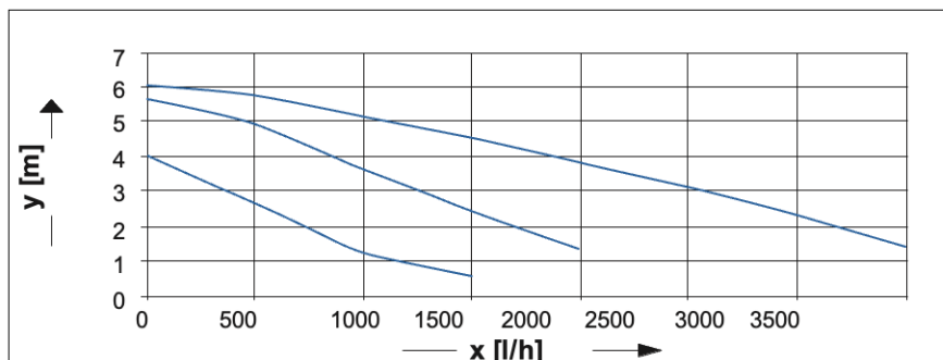
Рис. 16 Напір насоса на прикладі Wilo RS15/6
