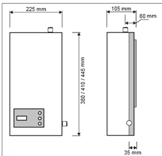
Рис. 5 Размеры отопительного котла AVL Joule AJ / AJ-S / AJ-WS / AJ-W
