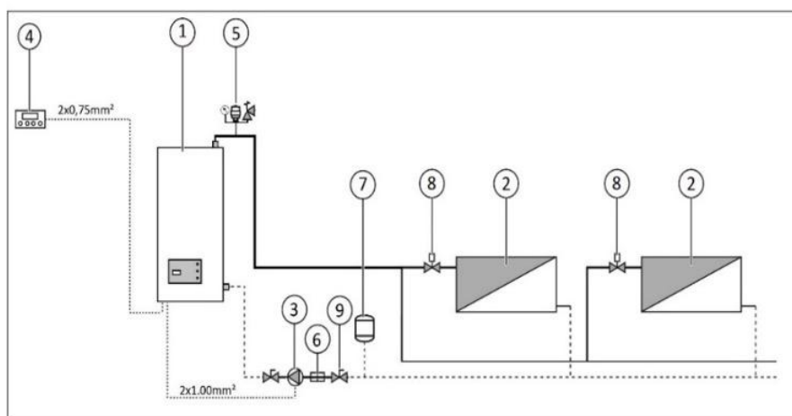
Рис. 17 Режим отопления и нагрева горячей воды в баке косвенного нагрева
