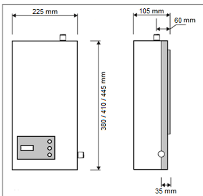
Рис. 5 Розміри опалювального котла AVL Joule AJ / AJ-S / AJ-WS / AJ-W
