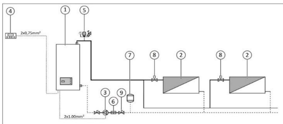
Рис. 17 Режим опалення та нагрівання гарячої води в баку непрямого нагріву
