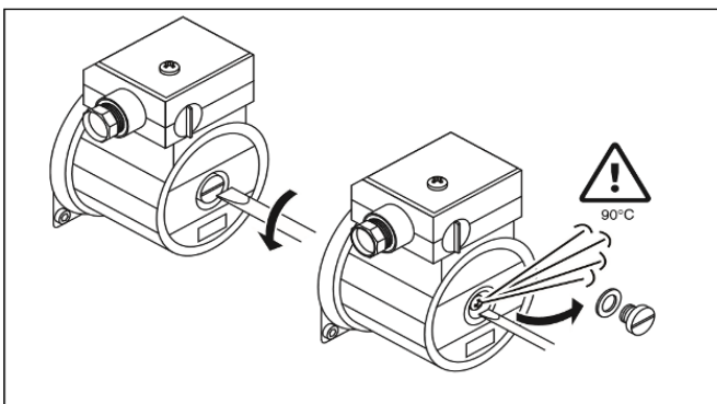
Рис. 8 Ослабление винта для спуска воздуха и проверка свободного хода
