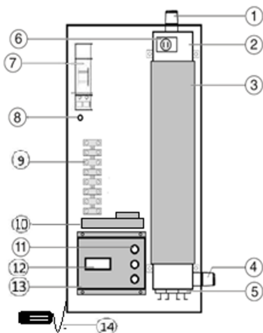
Рис. 4 Функціональні елементи котла AVL Joule AJ-W 3-9 кВт
