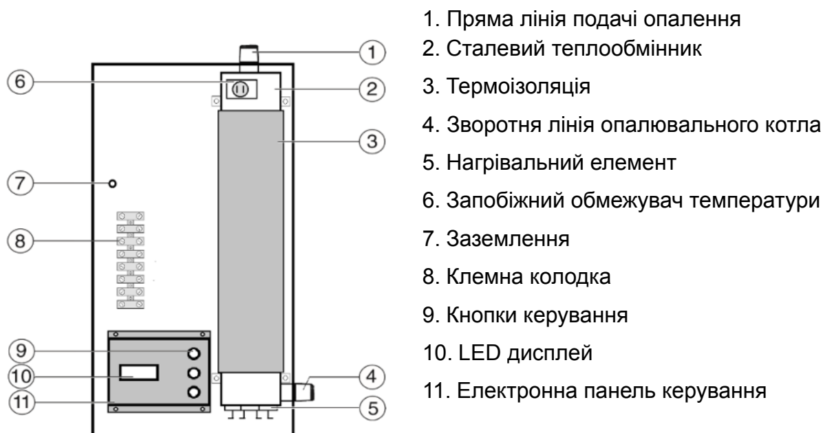
Рис. 1 Функціональні елементи котла AVL Joule AJ 3-9 кВт
